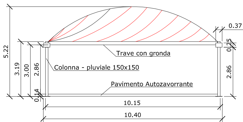
- PROSPETTO
