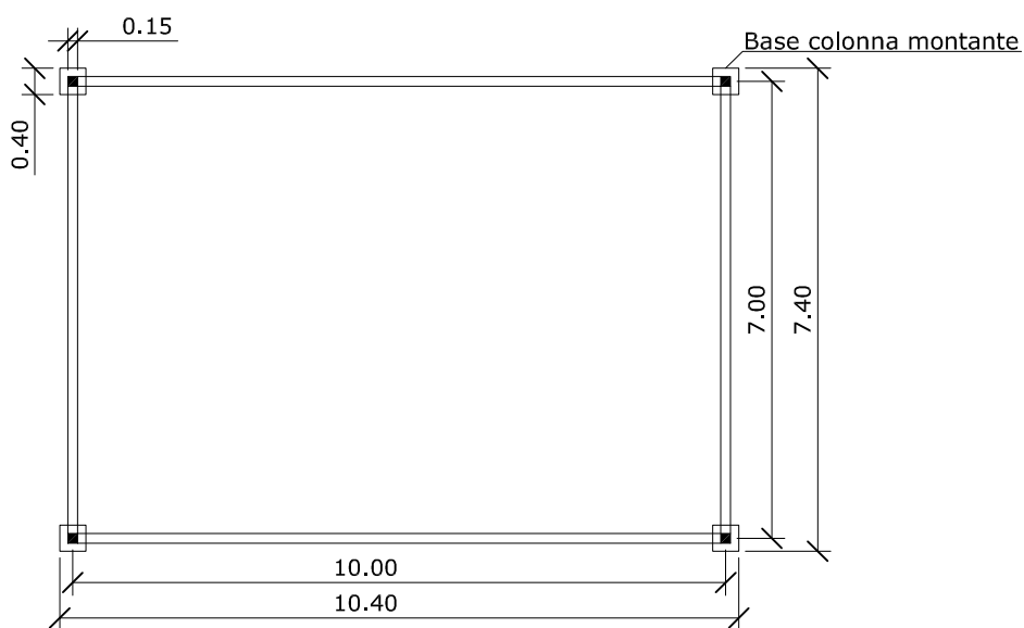
- PIANTA
